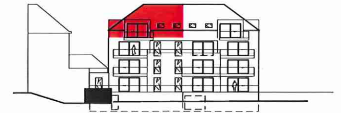
ACHTERGEVEL 2A
