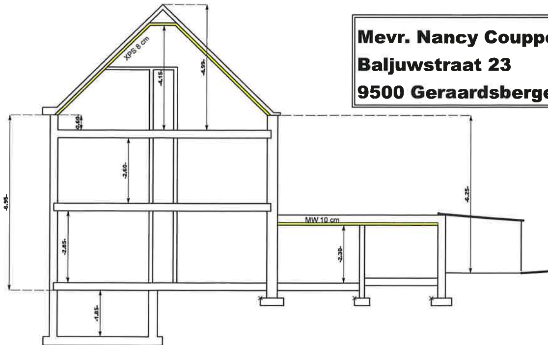
Dwarsdoorsnede
