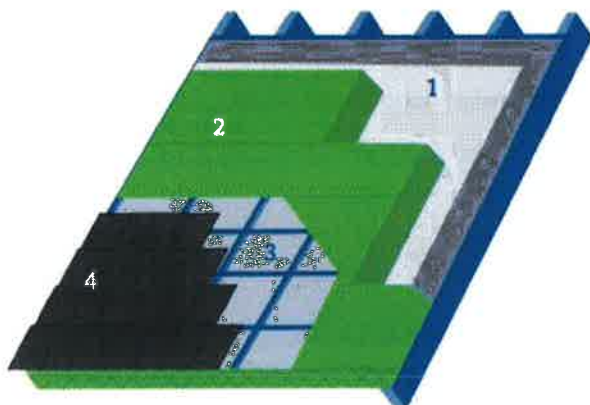
1. Dampschermbaan | 2. Isolatie | 3. Onderdak | 4. Dakbekleding
