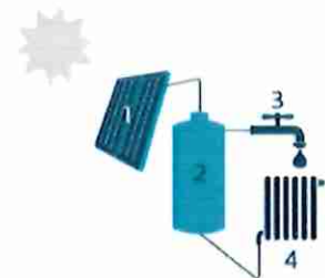
1 Zonnecollector | 2 Opslagvat zonneboiler | 3 Sanitair warm water | 4 Alditte element voor ruimteverwarming (optieeel)
